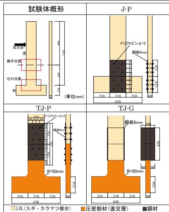
図 1 試験体概要図
