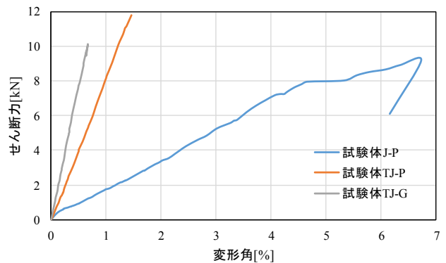
図 2 せん断力-変形角関係の包絡線
