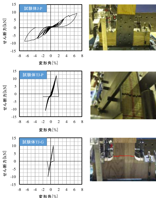
図2 せん断力-変形角関係と最大荷重時の様子
