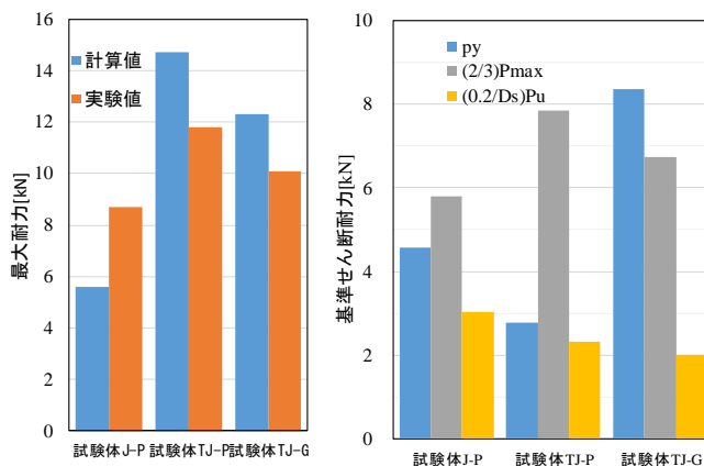
図4 実験値と計算値の比較 図5 基準耐力の比較
