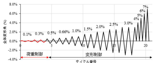
図-6 加力サイクル
