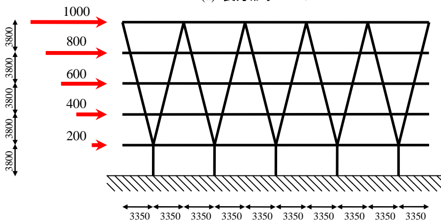
(b) 斜め柱ラーメン
