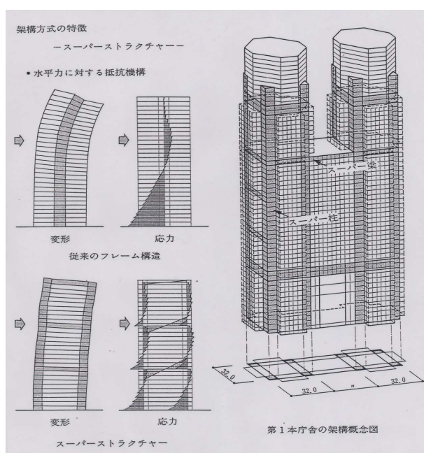
図 5.7 東京都庁舎第一本庁舎の構造計画
