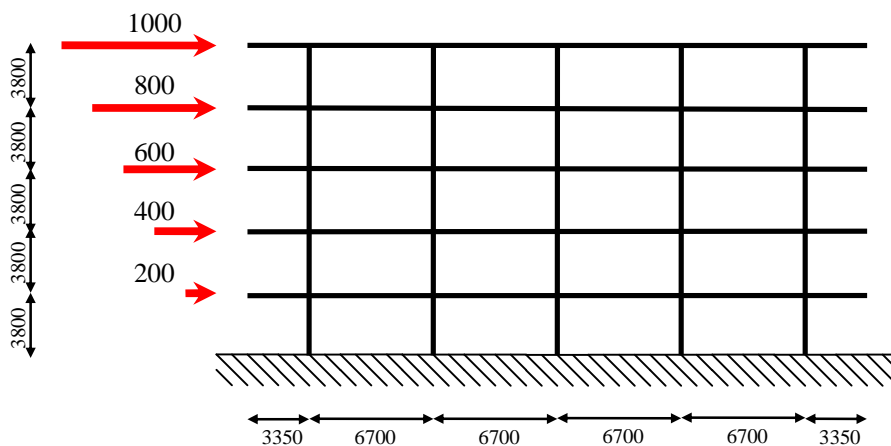
(a) 長方形ラーメン
