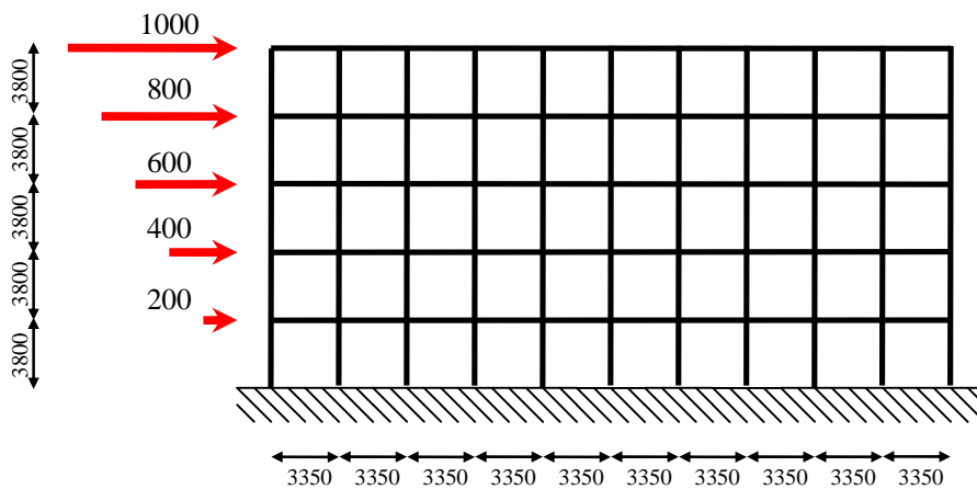
(c) チューブ架構
