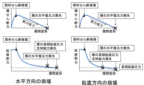
鉛直方向の崩壊: 水平復元力喪失変形角 > 層の長期鉛直応力支持能力喪失変形角 水平方向の崩壊: 層の長期鉛直応力支持能力喪失変形角 > 水平復元力喪失変形角
