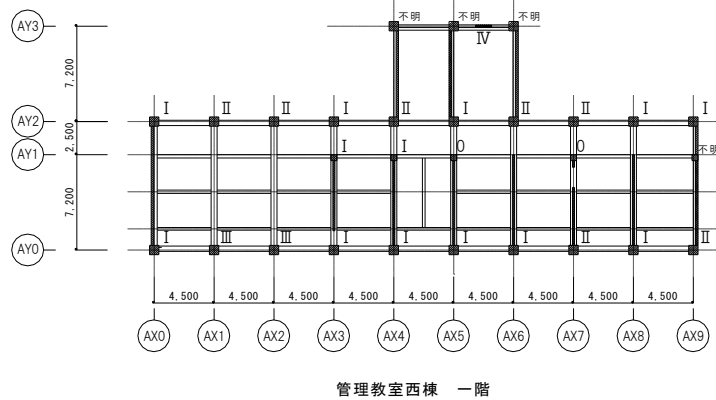
図7 管理教室西棟1階伏図と柱・壁の損傷度
