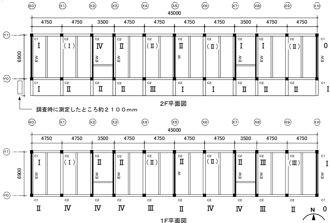
図4 柱梁伏図と柱の損傷度
