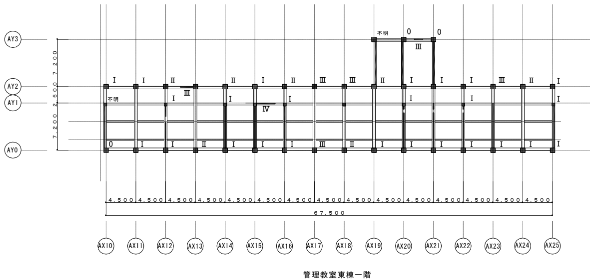
図6 管理教室東棟1階伏図と柱・壁の損傷度
