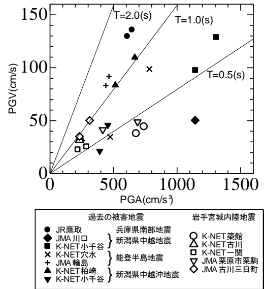
図2 最大加速度(PGA)－最大速度(PGV)
